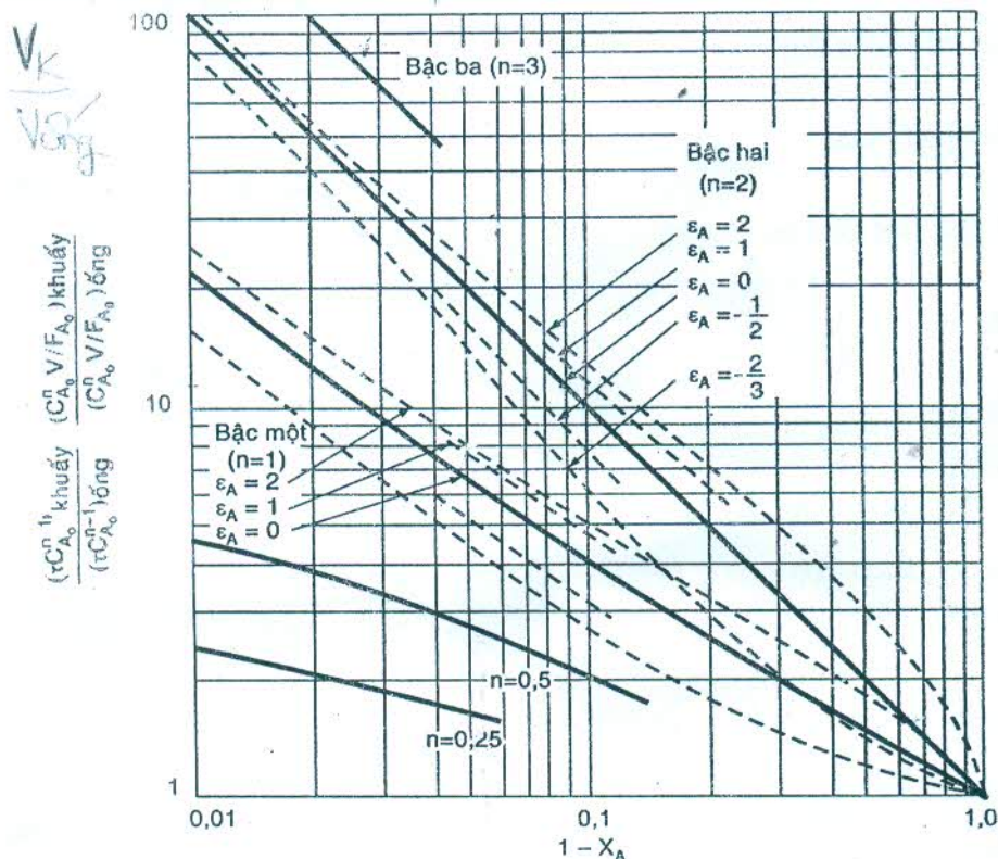
Hình 4.1: So sánh sự hoạt động của bình khuấy hoạt động ổn định và thiết bị phản ứng dạng ống cho phản ứng bậc n . Trục tung cho tỉ số V_k/V_\delta với cùng điều kiện nhập liệu
